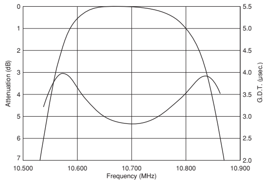
SFELF10M7FAB0-B0
