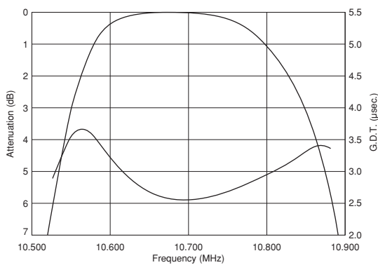
SFELF10M7FA00-B0
