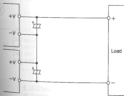
図9-1 出力電圧積み重ね直列運転
