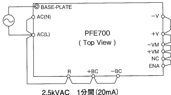
図16-1 入カースペースプレート間耐電圧試験方法
