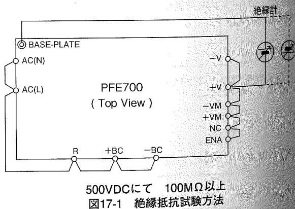
図17-1 絶縁抵抗試験方法
