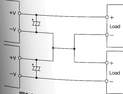
図9-2 正出力使用の直列運転
