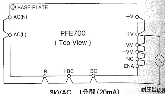
図16-2 入カ-出力間耐電圧試験方法
