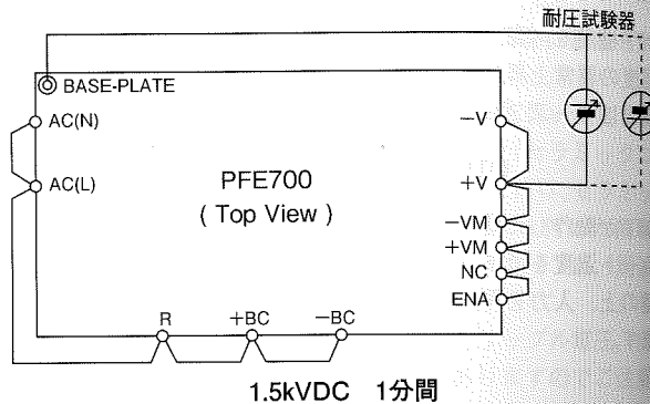
図16-3 出カースペースプレート間耐電圧試験方法
